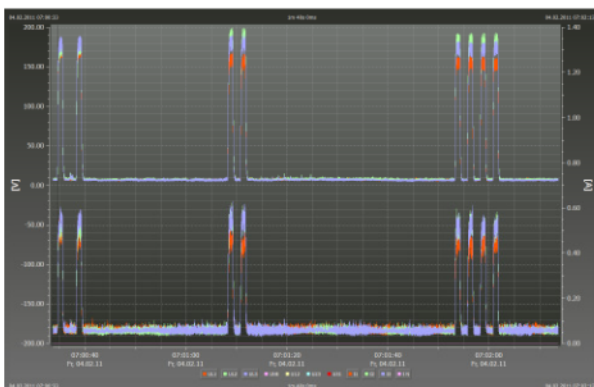
Telegrama de telemando de corrientes y tensiones
